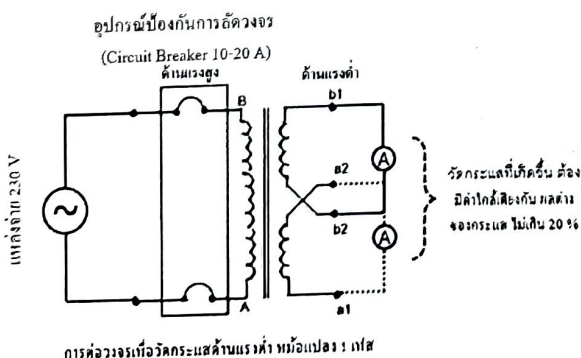
การต่อวงจรเพื่อวัดกระแสลัดวงจรด้านแรงต่ำ หม้อแปลง 1 เฟส
