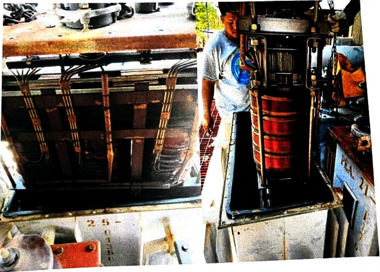
รูปภาพหม้อแปลง TR๒๕-๐๐๑๓๕๐ ๑๐๐KVA
