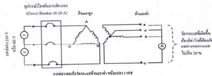
การต่อวงจรเพื่อวัดกระแสด้านแรงต่ำ หม้อแปลง 3 เฟส
